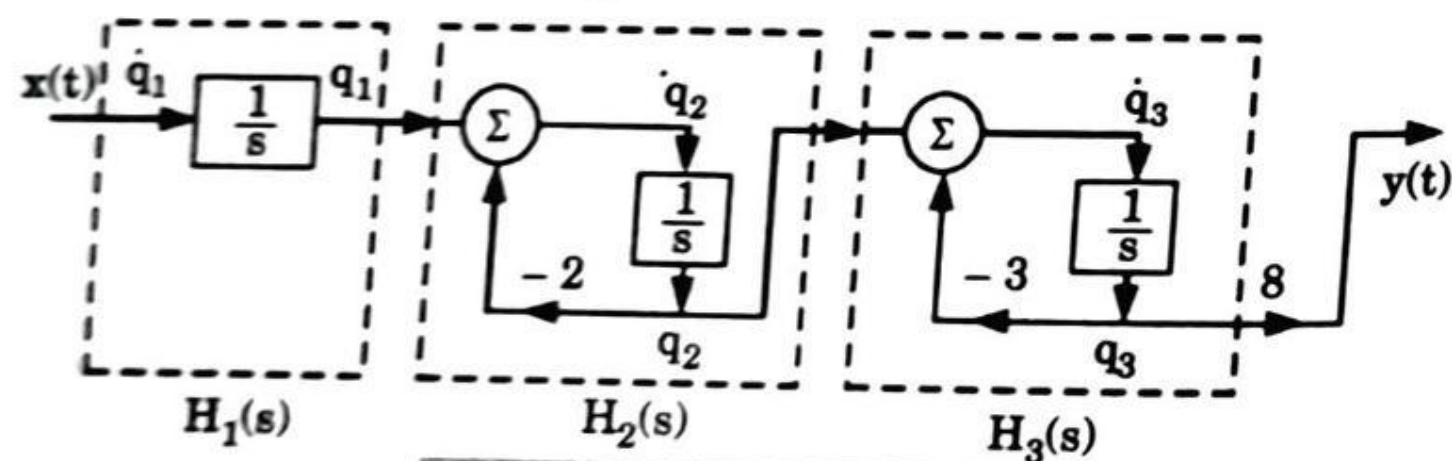
Fig. 4.10.1. Cascade form.
