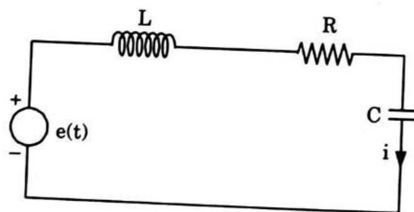
Fig. 1.25.2. Force-voltage analogous circuit.
