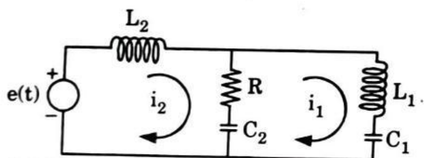
Fig. 1.31.2. Force-voltage analogous circuit.
