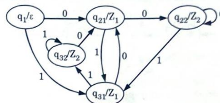
Fig. 1.36.1. Moore machine.
