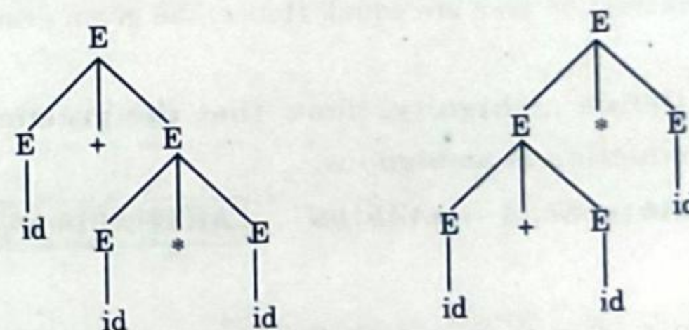
Fig. 3.13.1. Ambiguous grammar.
